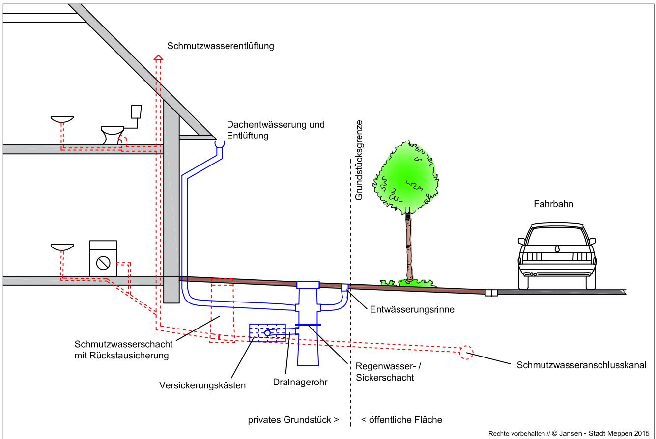
Skizze A - Musterschnitt EFH - ohne Maßstab
